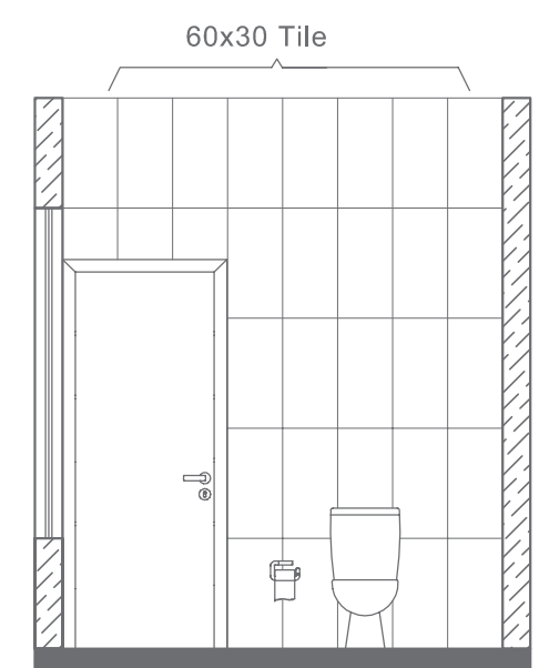
ELEVATION B
