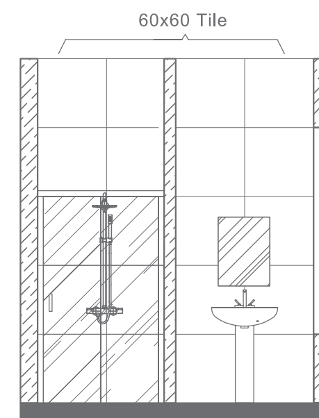
ELEVATION A
